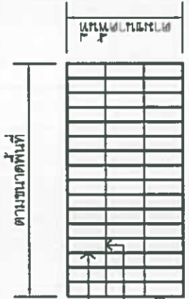
แบบขยายฝายตะแกรงเหล็ก Scale 1:20
